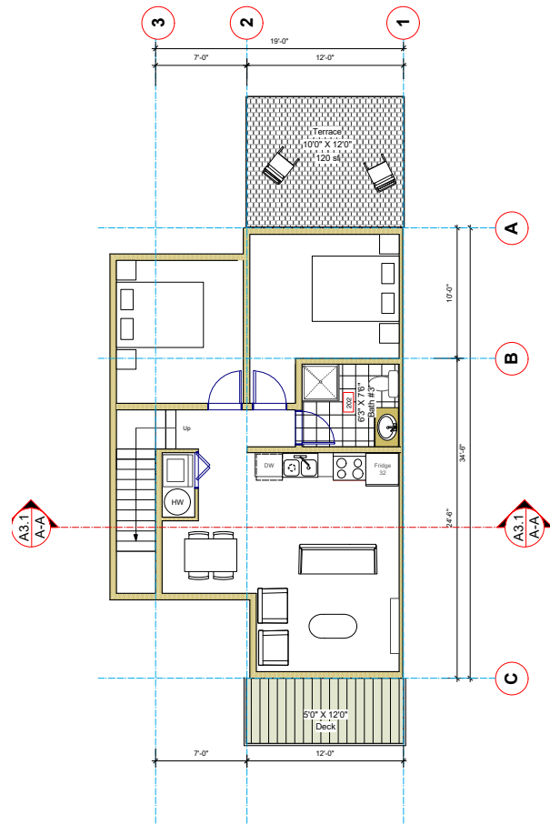
UNIT A2
